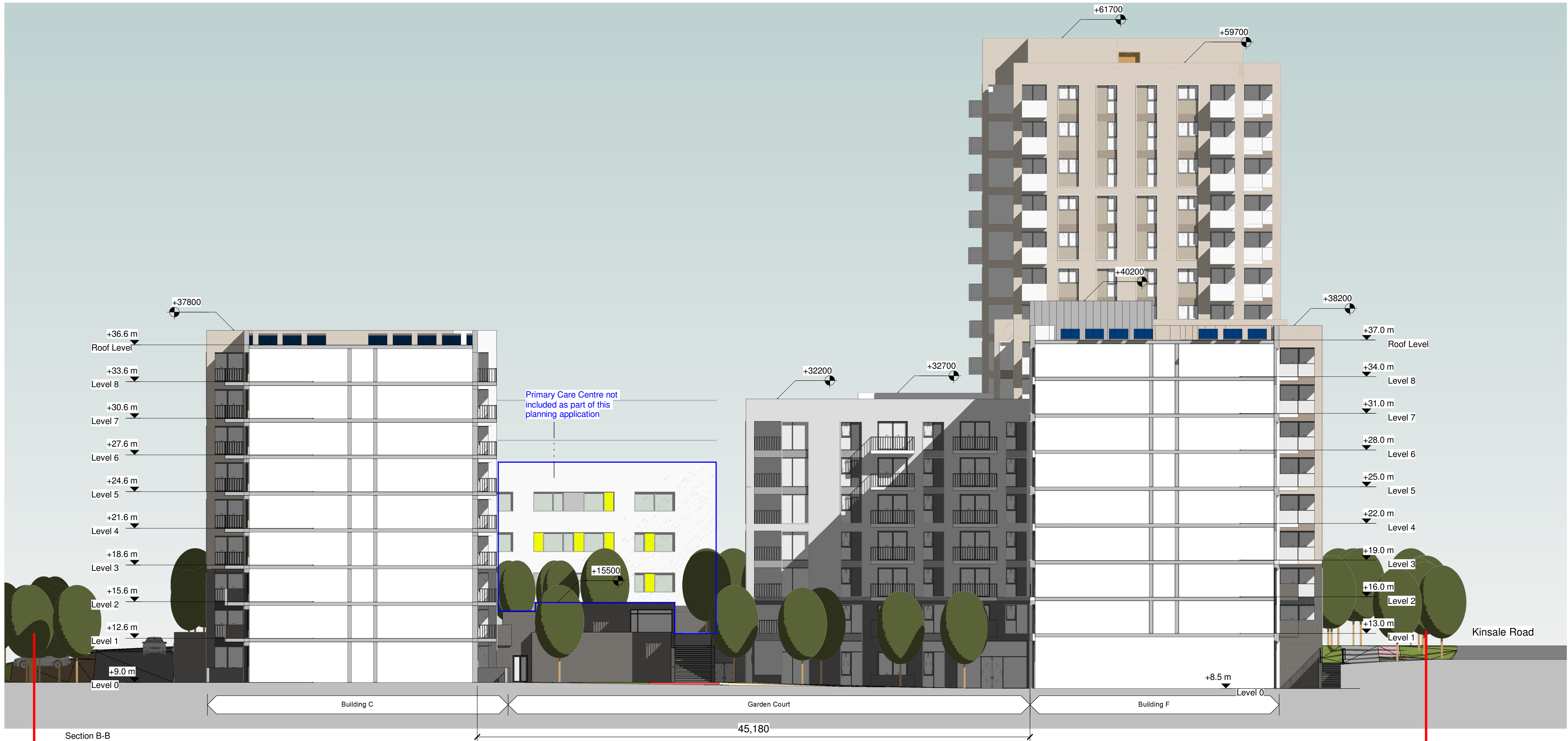
Section B-B 1 : 200
